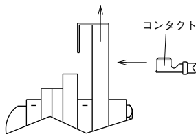
コンタクト保持具 開状態図
