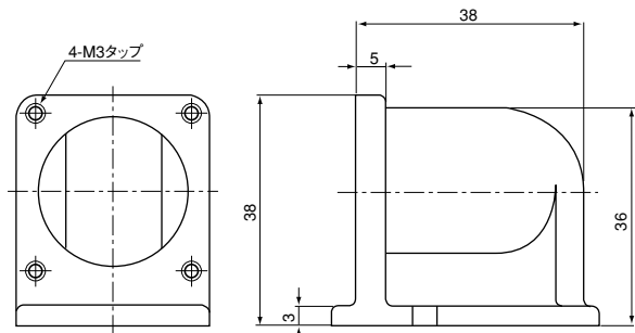
NJC-24用Lザ(座) (使用方法は7ページ参照)
