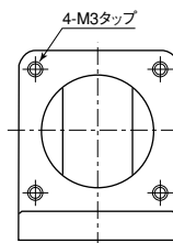
NJC-20用Lザ(座) (使用方法は7ページ参照)
