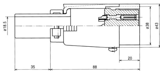
T-48*-PF
