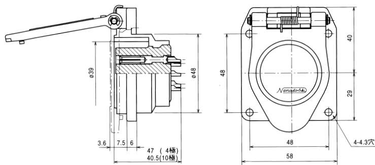
T-48*-RF
