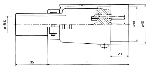
T-48*-PM
